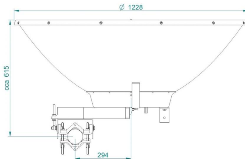
Fig.1 Dimensiones de la antena
